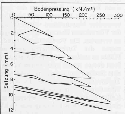
Bild 7. Grossbelastungsversuch: Last-Setzungsdiagramm
