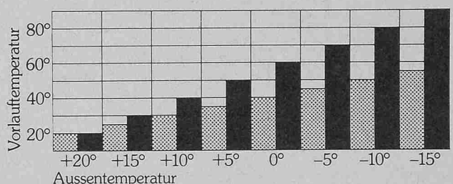
Vorlauftemperaturen bei einer Niedertemperaturheizung (Berechnungsgrundlage 55/45^{\circ}\text{C} ) und einer konventionellen Radiatorenheizung bei unterschiedlichen Aussentemperaturen. Ablesbeispiel: Bei einer Aussentemperatur von -5^{\circ}\text{C} beträgt die Vorlauftemperatur bei der NTR-Heizung 45^{\circ}\text{C} , bei der konventionellen Radiatorenheizung 70^{\circ}\text{C} . Punktierter Balken: NTR-Heizung. Schwarze Balken: Konventionelle Radiatorenheizung
