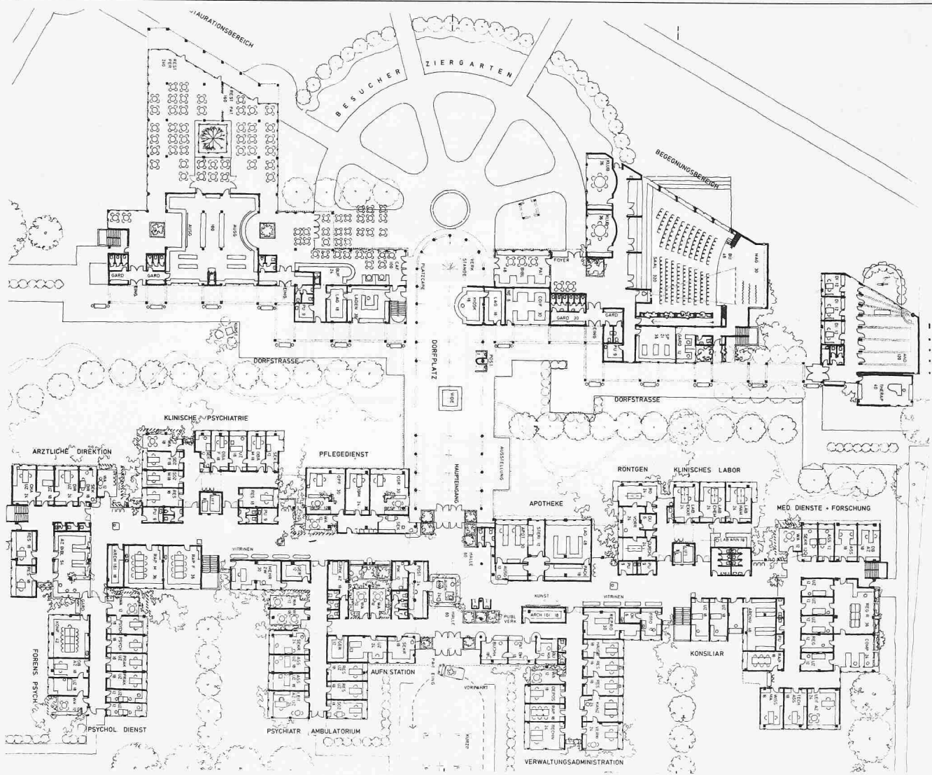
Grundriss Erdgeschoss 1:800
