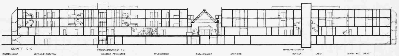
Schnitt C-C 1:800
