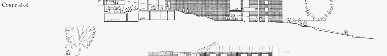
Façade sud-ouest
