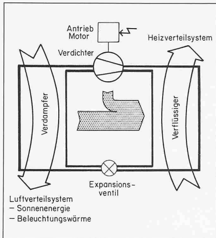
Bild 8. Wärmepumpe
