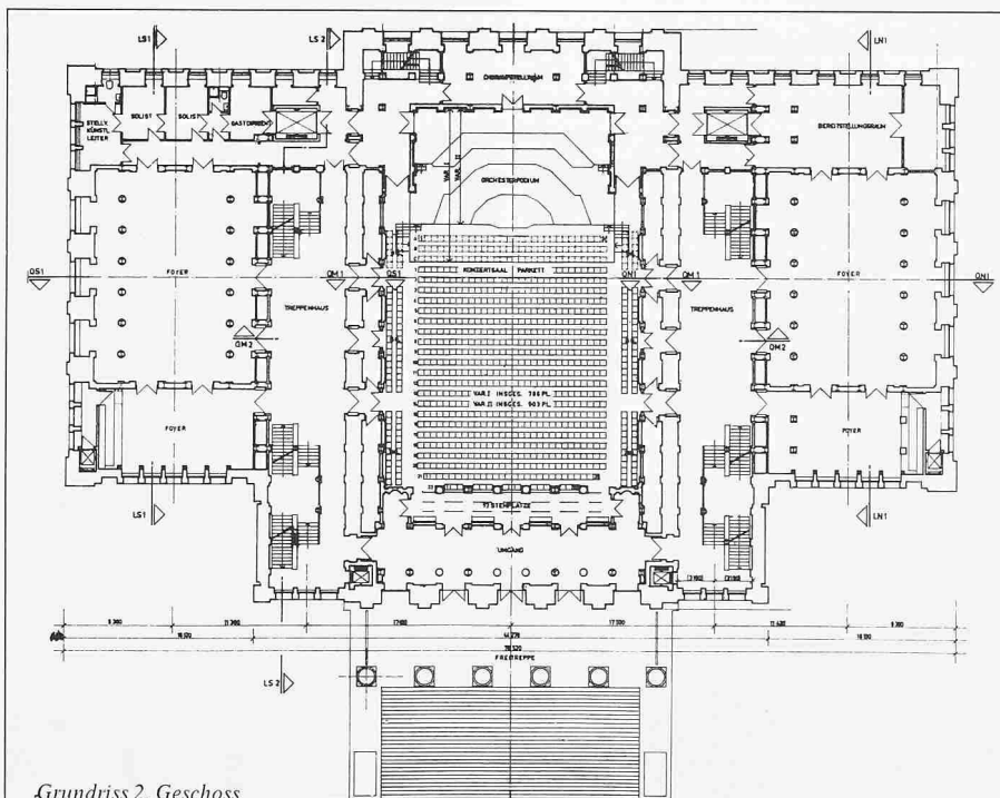
Grundriss 2. Geschoss
