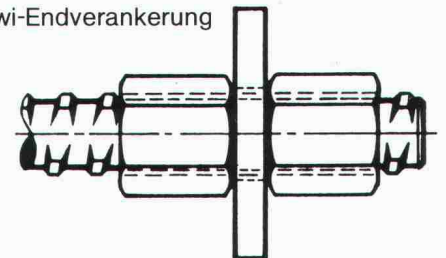
Gewi-Endverankerung
