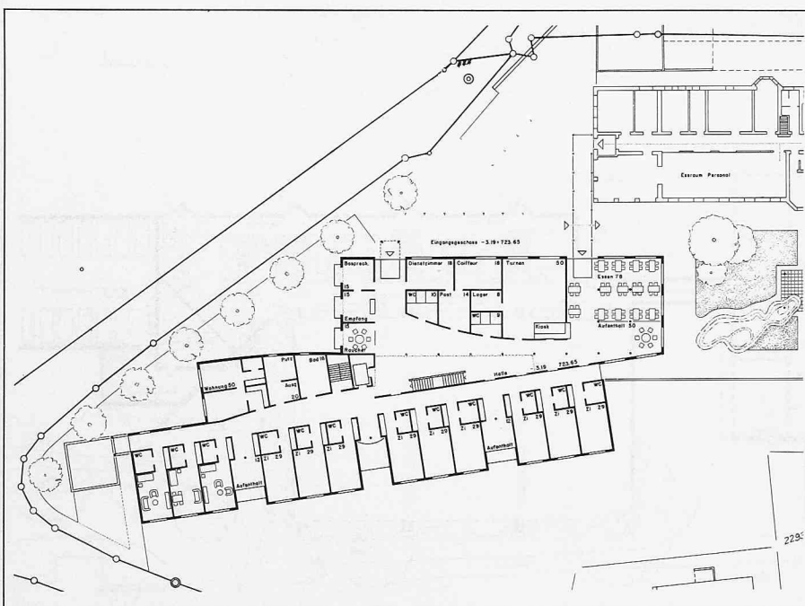
Lageplan 1:1600
