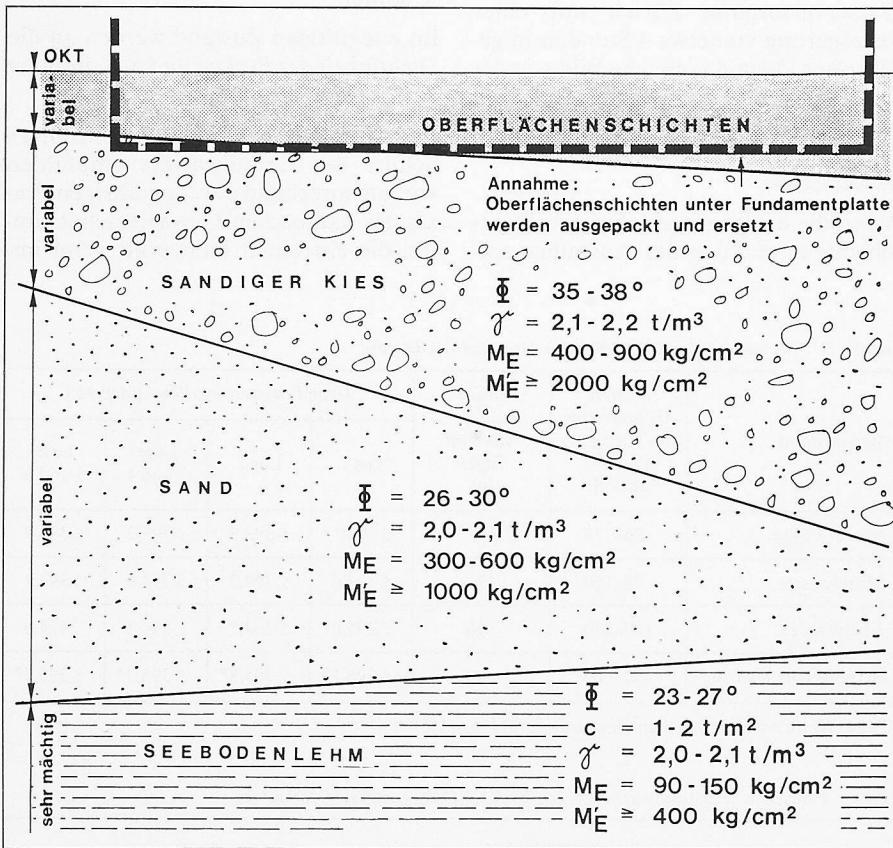
Bild 3. Baugrundmodell
