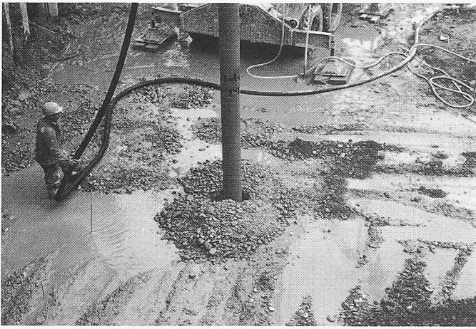
Bild 6. Rüttelverdichtung
