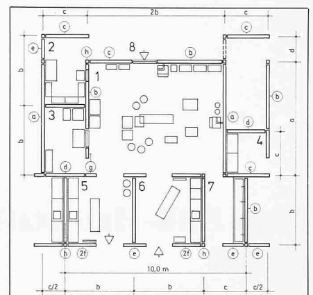
Bild 18. OP-Funktionseinheit (quadratisch), Bestandteil der Grundrissvariante im Bild 15, 1 Operationsraum, 2 Schaltraum, 3 Messraum, 4 Lagerraum (z. B. Schienen-), 4a Substerilisation, 5 Ausleitung/Entsorgung, 6 Einleitung, 7 Waschraum Ärzte, 8 Versorgung - reine Güter
