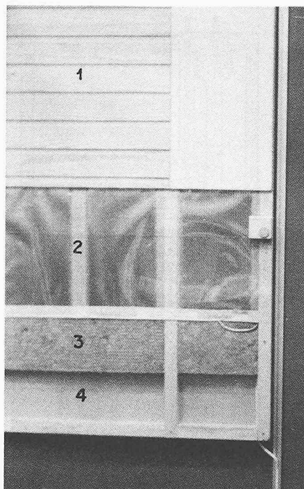
Elektrische Heizfolie. 1 Innenraum-Holztäfer, 2 Heizfolie, 3 Wärmedämmung, 4 Mauerwerk
