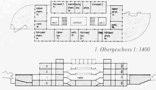
Schnitt 1:1400
