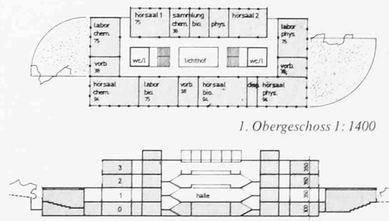
Schnitt 1:1400
