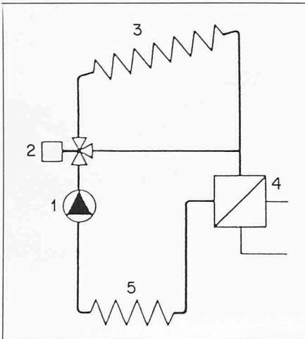
Kombination Luftregister/Erkolloktor 1 Umwälzpumpe 2 Verteilventil 3 Luftregister Carport 4 Verdampfer, Wärmepumpe 5 Erkolloktor
