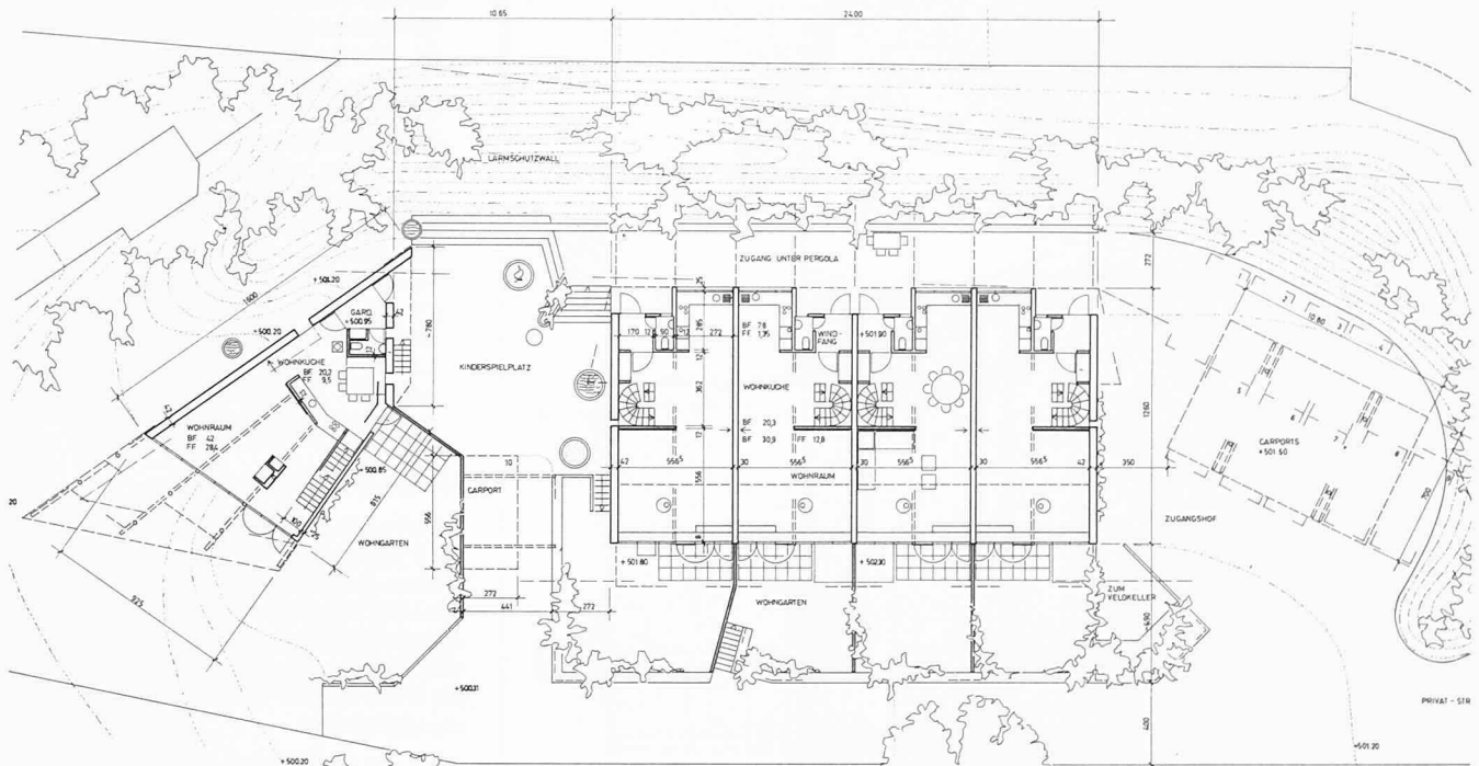
Grundriss, Erdgeschoss
