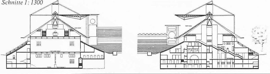
Schnitte 1: 1300
