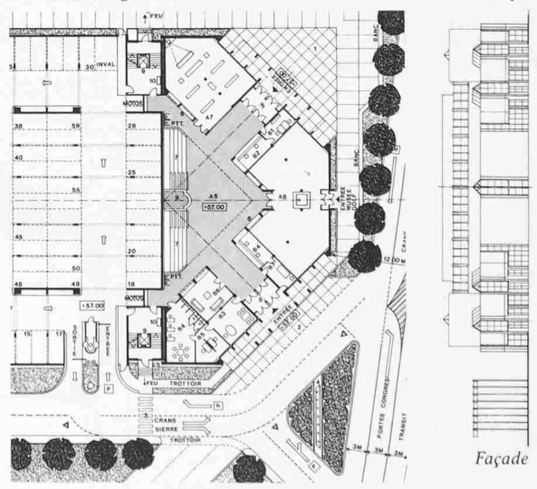
Maison de congrès, niveau entrées
