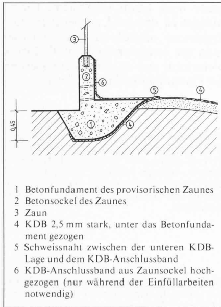
Bild 4. Anschluss der Kunststoff-Dichtungsbahn an den provisorischen Zaun während der Einfüllarbeiten
