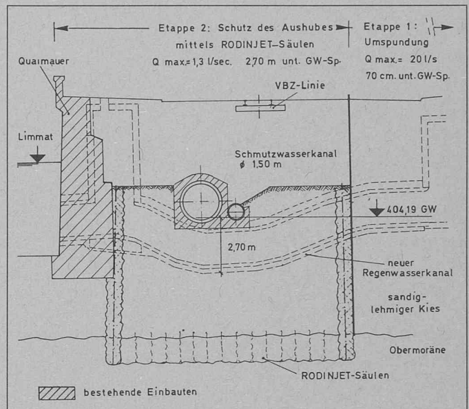
Zürich, Neumühlequai. Neuer Regenwasserkanal (Längsschnitt), Schmutzwasserkanal (Querschnitt)
