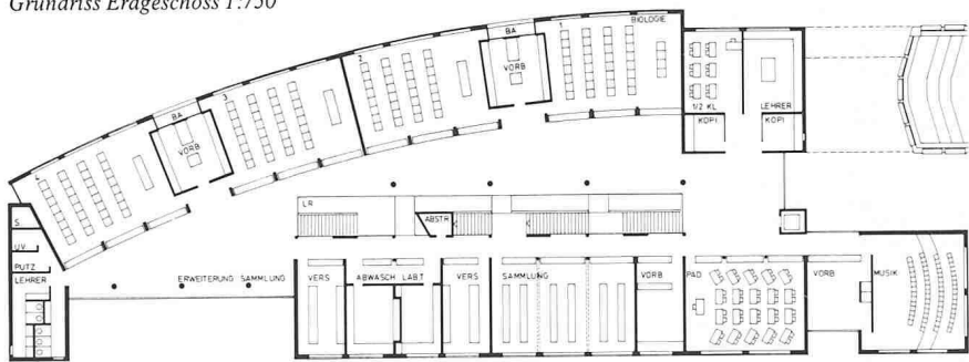
1. Obergeschoss
