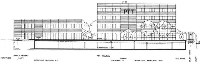
Schnitt B-B
