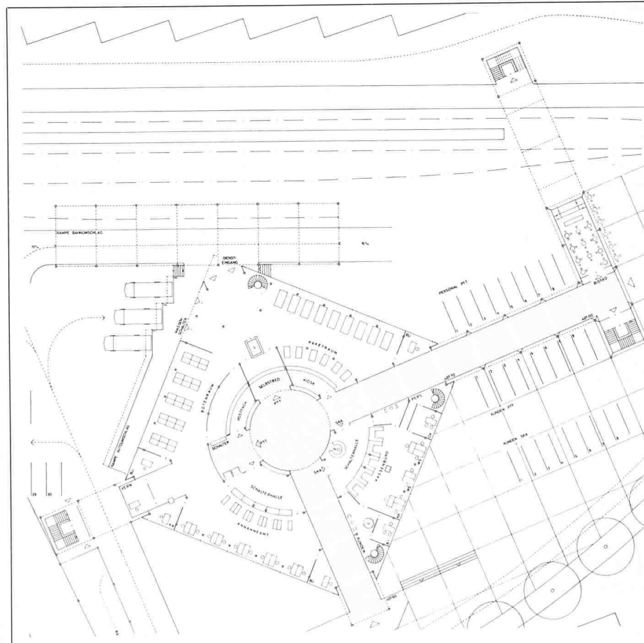
Grundriss Erdgeschoss 1:800
