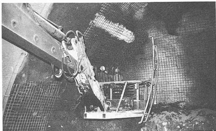
Bild 8. Befestigung der Bewehrungsmatten. Die weisse Zone oberhalb des Arbeitskorbes entstand wegen eines naheliegenden Gefrierrohrs
