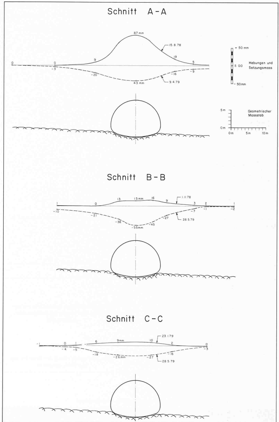
Bild 5. Hebungen und Setzungen im Querschnitt
