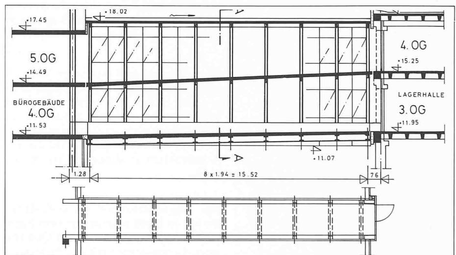
Bild 2. Längsschnitt und Grundriss der Passerelle
