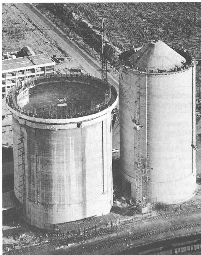
Bild 4 (rechts). Endphasen der Erstellung des ersten Tonerdesilomantels und der Hebung des Kokksilodaches
