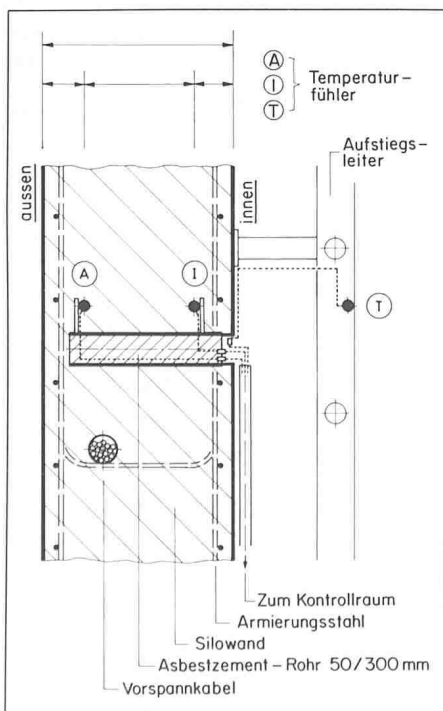
Bild 9(links). Schema einer typischen Temperatur-Messstelle in der Tonerdesilowand
