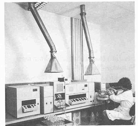
Direkte Luftabsaugung am Atomabsorptionsspektrometer, das zur Spektralanalyse dient
