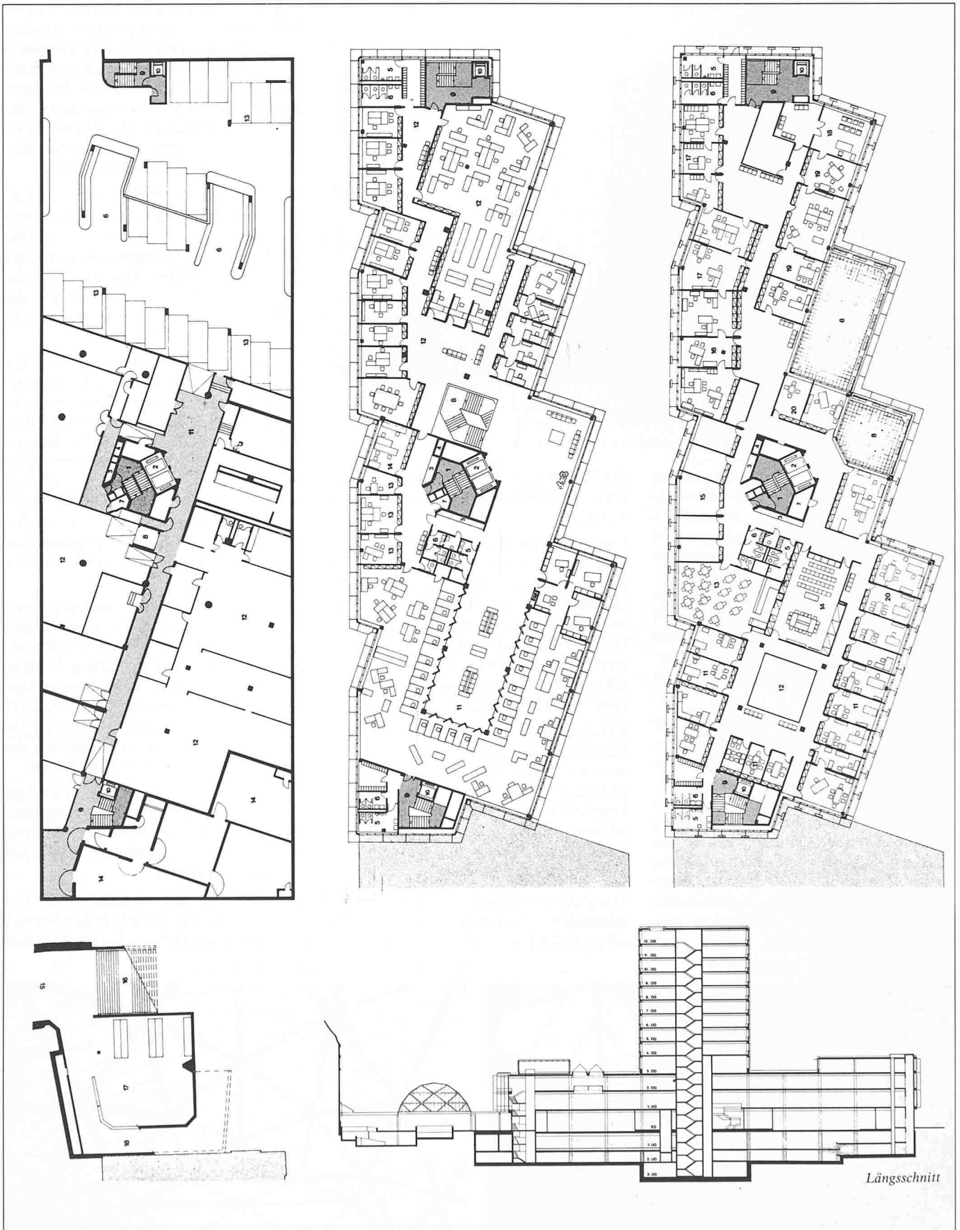
1. Untergeschoss. 1 Hochhaus-Sicherheitstrep- ppenhaus, 2 Hochhauslift, 3 Installationen, 4 Hei- zungskamine, 5 Parkgarage Einfahrt, 6 Verbindun- gen 2. UG, 7 Putzraum, 8 Transportlift EG-1. UG, 9 Nebentreppen, 10 Nebenlift, 11 Verbindungsgang, 12 Rechenzentrum, 13 Parkfelder, 14 Schutzräume, 15 SBB-Unterführung Ost, 16 Treppe Unterführung Ost, 17 Schliessfächer, 18 Fussgängerrampe
