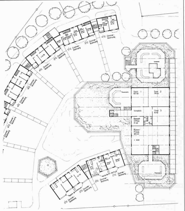
1. Obergeschoss
