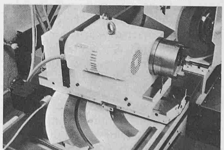
Bild 3. Werkzeuggestisch mit Schwenkeinheit
