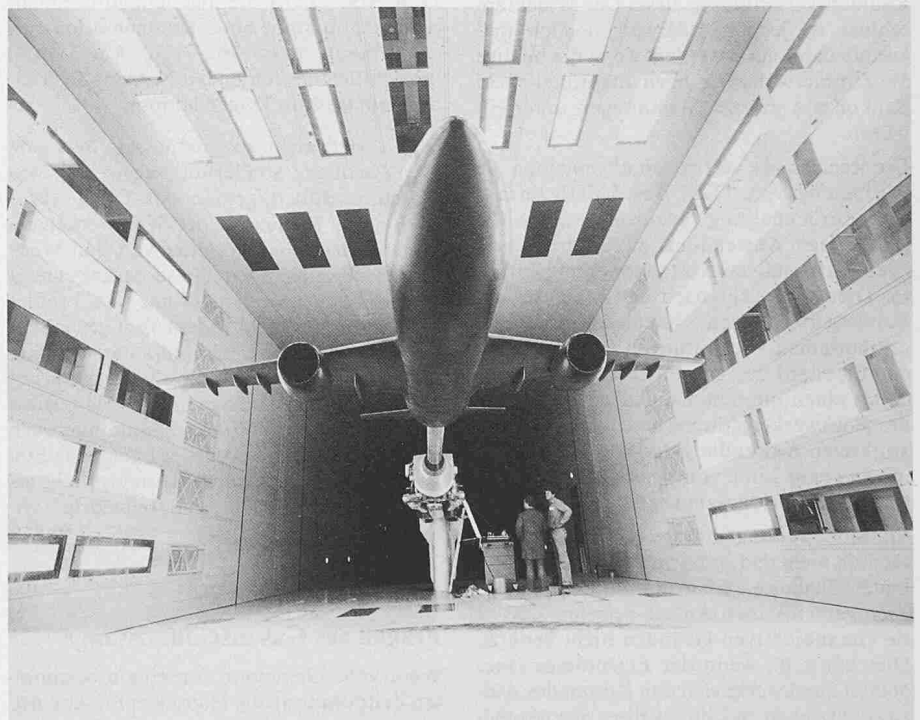
Ein massstabgerechtes Airbus-A300-Modell am Heckstiel-Modellträger, mit dem jede gewünschte Lage im Luftstrom gesteuert werden kann
