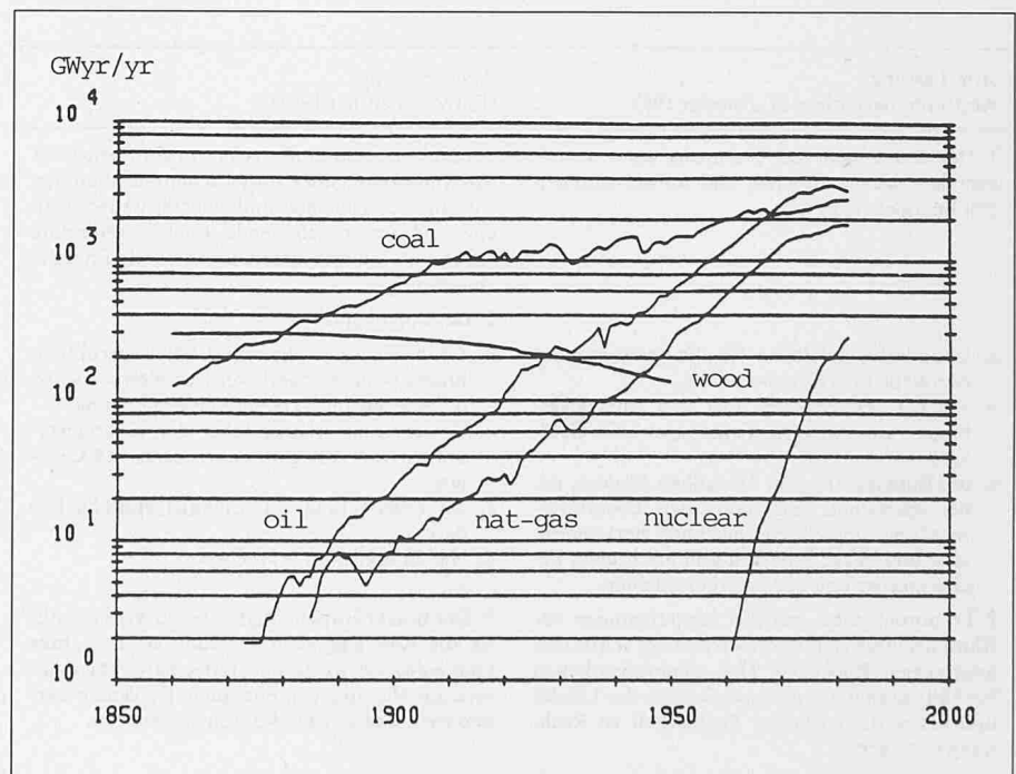
Bild 1. Entwicklung des Weltprimärenergieverbrauchs (Grübler und Nakicenovic, 1987). Globaler Verbrauch verschiedener Primärenergieträger (Holz, Kohle, Erdöl, Erdgas und Kernenergie) in GW-Jahren pro Jahr (ein GW-Jahr entspricht etwa einer Million Tonnen Steinkohleeinheiten). Im logarithmischen Massstab können die unterschiedlichen Wachstumsraten einzelner Energieträger bzw. deren Veränderungen deutlich abgelesen werden. Diese unterschiedlichen Wachstumsraten führen zu Veränderungen im Marktanteil einzelner Energieträger.
