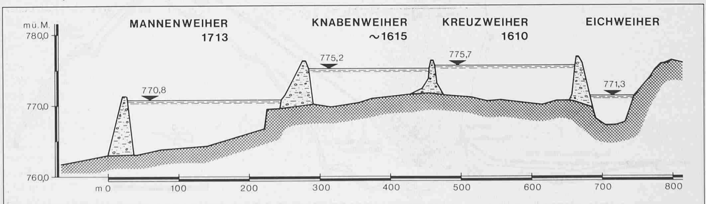
Bild 5. Zehnfach überhöhtes Längsenprofil durch die Weiher auf Dreilinden in St. Gallen SG
