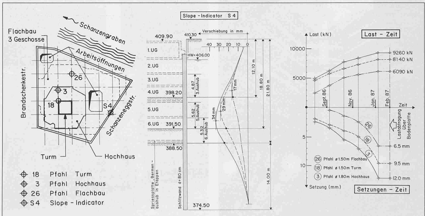
Gegenüberstellung von Lastaufbringung und Pfahlsetzungen für drei unterschiedlich belastete Pfähle. Bis zur Lastabtragung über die Bodenplatte erreicht die max. Setzungsdifferenz den Betrag von 5.5 mm
