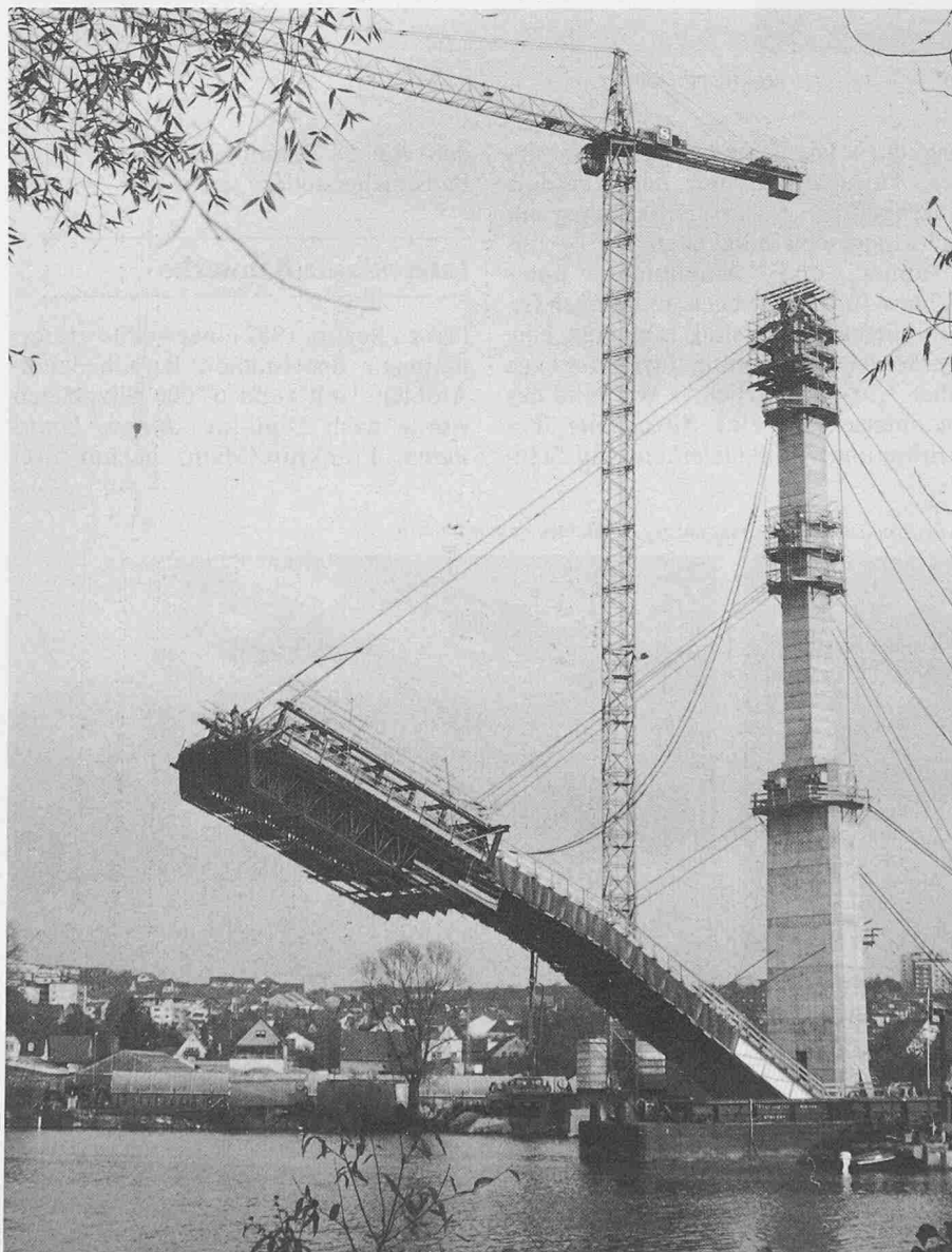
Bild 8. Zweigleisige Eisenbahnbrücke in Veitshöchheim für die Neubaustrecke Hannover-Würzburg. Herstellen des Bogens im Freivorbau mit Abspannungen zu Hilfspylonen.
