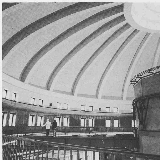
Bild 6. Kuppelbau eines alten Pumpwerkes in Duisburg vor (a) und nach der Instandsetzung der Stahlbetonninnenseite (b)
