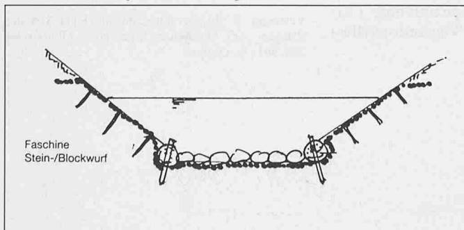
Bild 25. Vollständige Bachauskleidung
