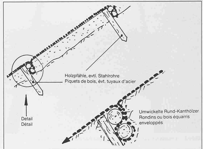
Bild 15. Befestigung von Geotextilien bei grossen Kräften
