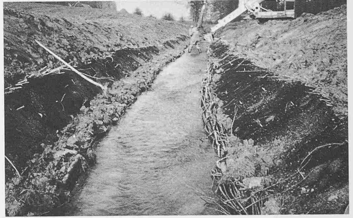
Bild 8. Befestigung von Grünufeln; Aufgabe des Geotextils: Stützen und Festigen der Oberflächenschicht und des Wurzelwerks; Geotextilart: feinporig, hohe Festigkeit; Funktionsdauer: im allgemeinen permanent, evtl. nur kurzfristig bis zur ausreichenden Durchwurzelung
