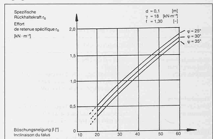
Bild 17. Spezifische Rückhaltekräft in Abhängigkeit von der Böschungneigung
