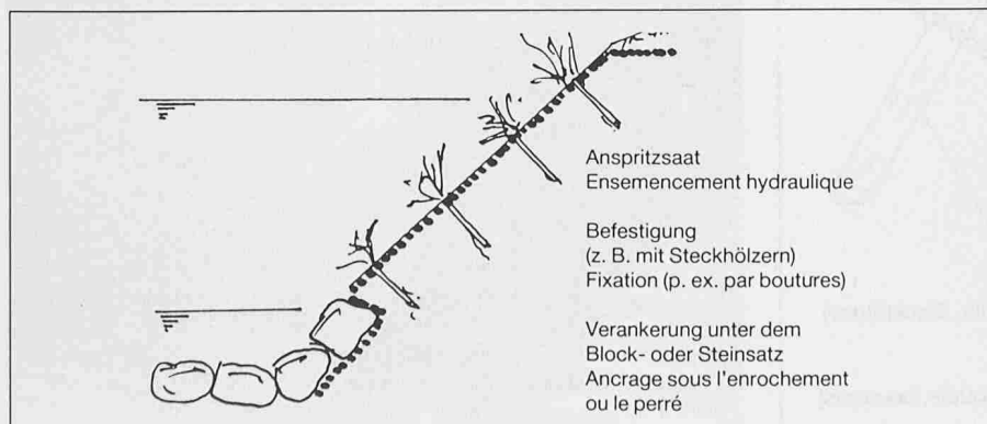
Bild 8. Befestigung von Grünufeln; Aufgabe des Geotextils: Stützen und Festigen der Oberflächenschicht und des Wurzelwerks; Geotextilart: feinporig, hohe Festigkeit; Funktionsdauer: im allgemeinen permanent, evtl. nur kurzfristig bis zur ausreichenden Durchwurzelung
