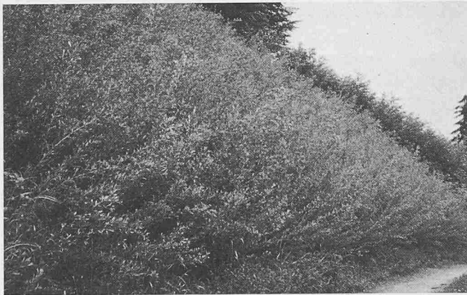
Bild 8. Befestigung von Grünufeln; Aufgabe des Geotextils: Stützen und Festigen der Oberflächenschicht und des Wurzelwerks; Geotextilart: feinporig, hohe Festigkeit; Funktionsdauer: im allgemeinen permanent, evtl. nur kurzfristig bis zur ausreichenden Durchwurzelung
