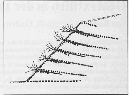
Bild 5. Aufbau einer begrünten geotextilarmierten Polsterwand; Begrünung: - Einbau von Busch- bzw. Heckenlagen; - Anspritzsaat auf Geotextiloberfläche; Aufgabe des Geotextils: Armieren des Erdkörpers, Filtern (Erosionsschutz an der Oberfläche); Geotextilart: feinporig, hohe Festigkeit; Funktionsdauer: permanent
