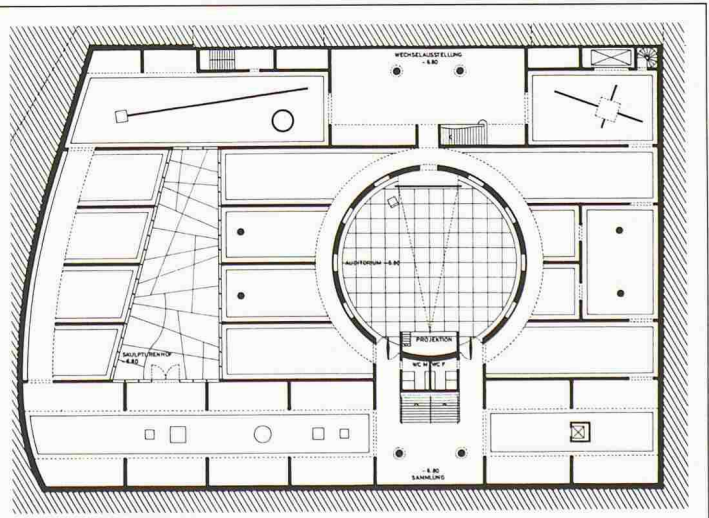
1. Untergeschoss
