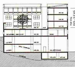
Querschnitt B-B
