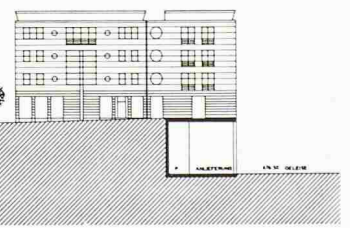
Ansicht von der Seite D-D
