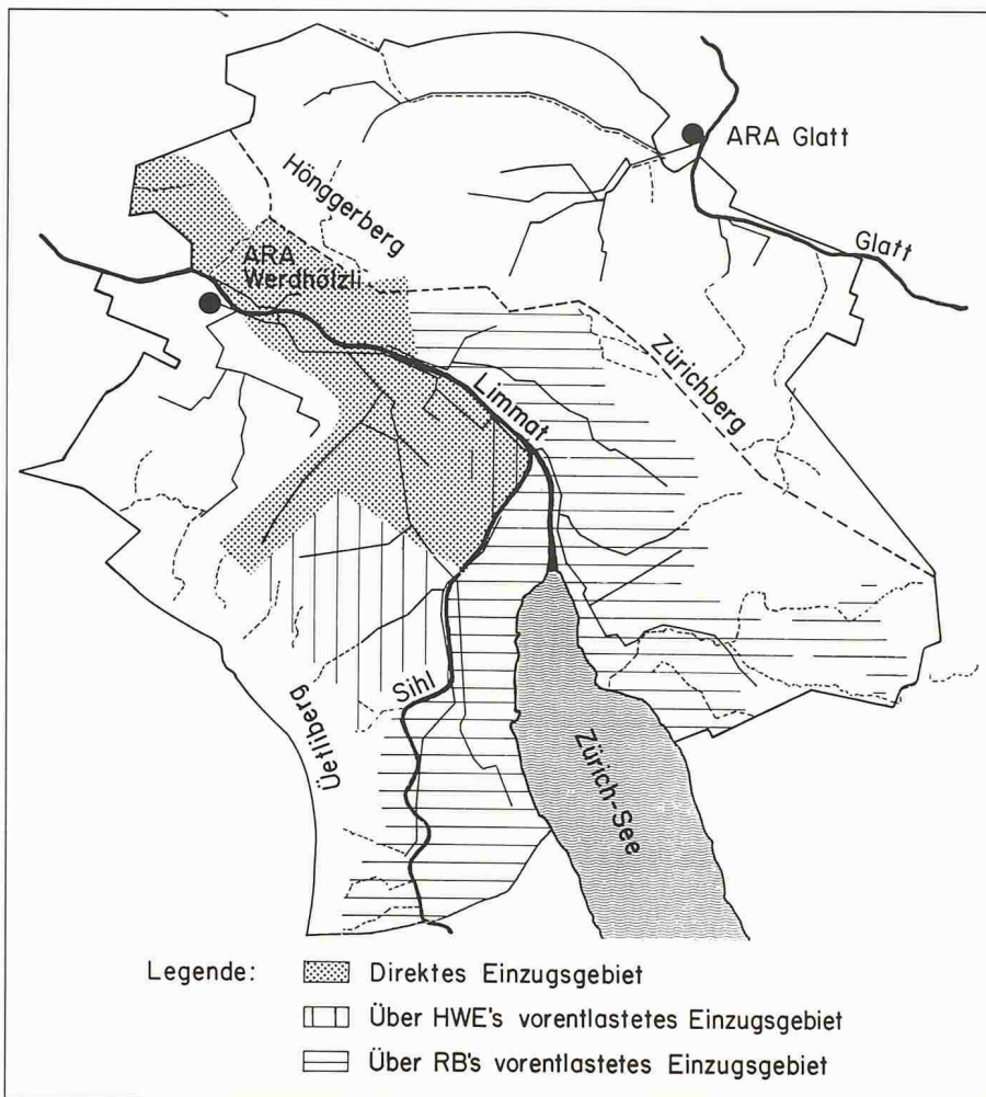
Bild 2. Das Einzugsgebiet des Regenbeckens auf der Werdingen
