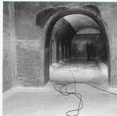
Wasserreservoir Muttentenzwald: Kombination von verschiedenen Sanierungs-Methoden: Injektionen gegen eindringendes Wasser und zur Verfestigung des Gewölbes, Auskleidung durch starre Abdichtung.
