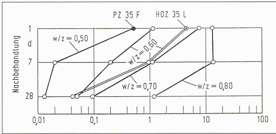
Bild 1. Zusammenhang zwischen Nachbehandlung, Wasser/Zement-Wert (W/Z), Zementart und dem spezifischen Permeabilitätskoeffizienten K (in 10^{-16} m^2 ) verschiedener Betone; Werte in Klammern = HOZ 35 L
