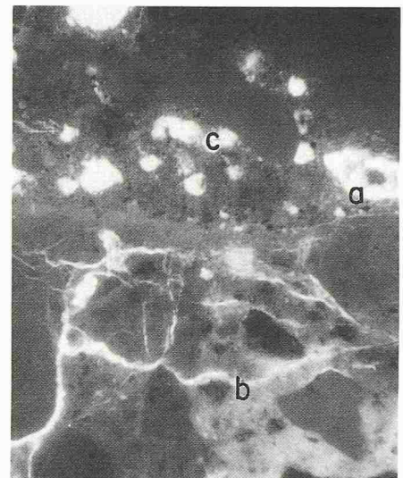
Bild 3. Übergangsbereich (a) zwischen Altbeton mit Rissen (b) und Sanierungsmörtel mit kugeligen Luftporen (c) (Gefügebildung, Fluoreszenzmikroskopie, Vergrößerung 46fach) (Hächler)
