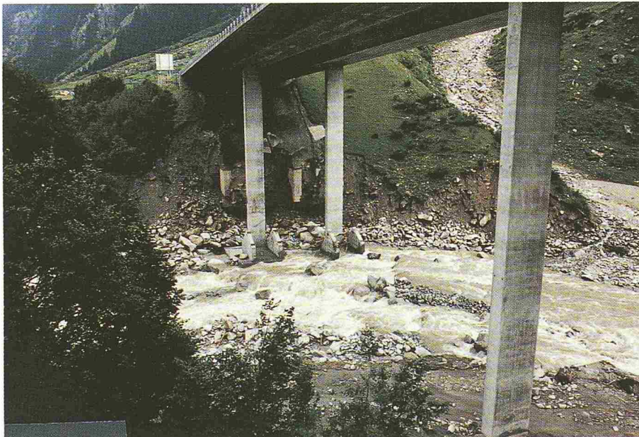
Bild 13. Rechtes Ufer beim Widerlager Nord, und Pfeiler B/G Bildautor: T.R. Schneider, 1878/25
