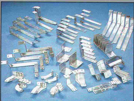
DIVERSE ANSCHLÜSSE Serienvorbindungen aus Kupfer verzinkt, vernickelt oder versilbert für Schalt- und Verteilanlagen.
