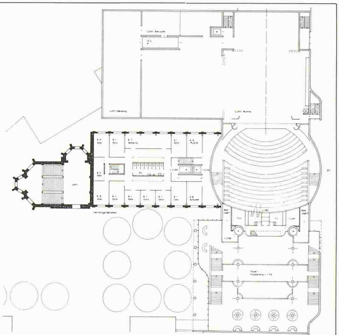
Parkett-, Bühnengeschoß
