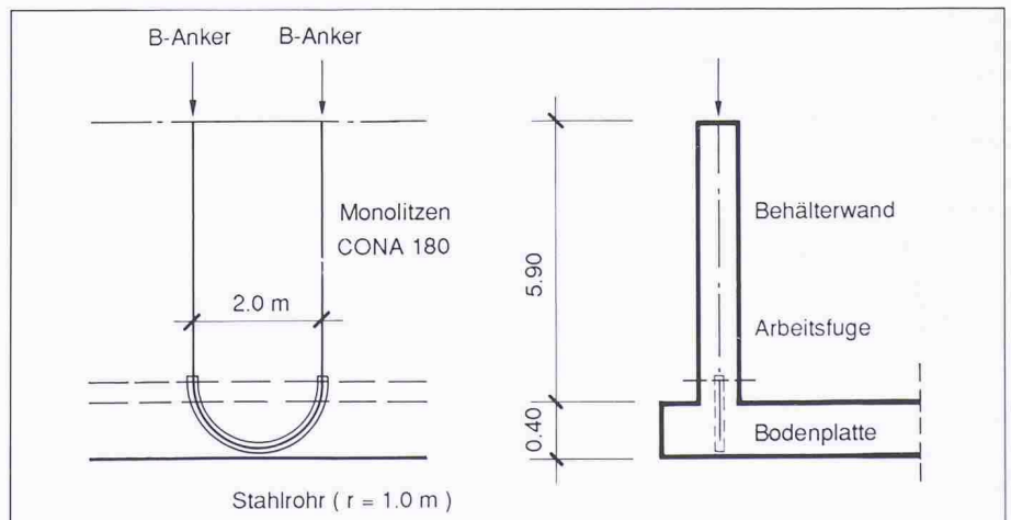
Bild 4. Prinzip der vertikalen Wandvorspannung
