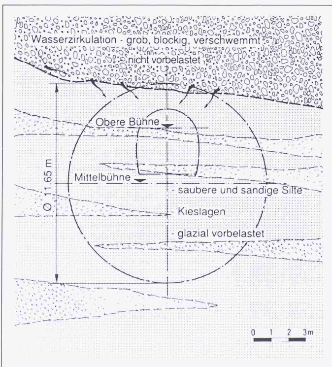
Bild 2. Bodenverhältnisse beim Schildhalt
