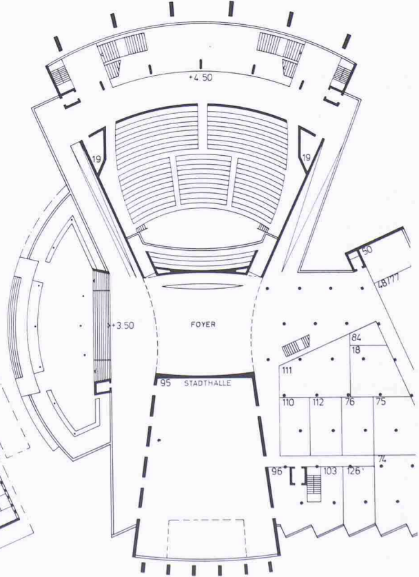
1. Obergeschoss
