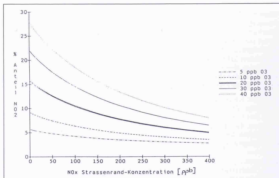
Bild 6. \text{NO}_2 -Anteil am Strassenrand (Volumenprozent, \text{NO}_2/\text{NO}_x in ppb); Jahresmittel; Windrichtung gleich verteilt; Autobahn; (nach [17])
