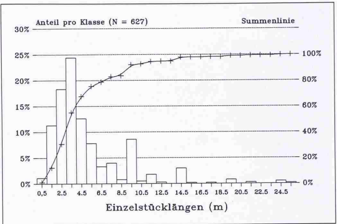
Bild 7. Längenverteilung von in Oberrammer Seitenbächen vorgefundenem Holz. Obschon aus seitlichen Rutschungen laufend neue Bäume ins Gerinne gelangen, ist der Hauptteil der Stücke kürzer als 6 Meter
