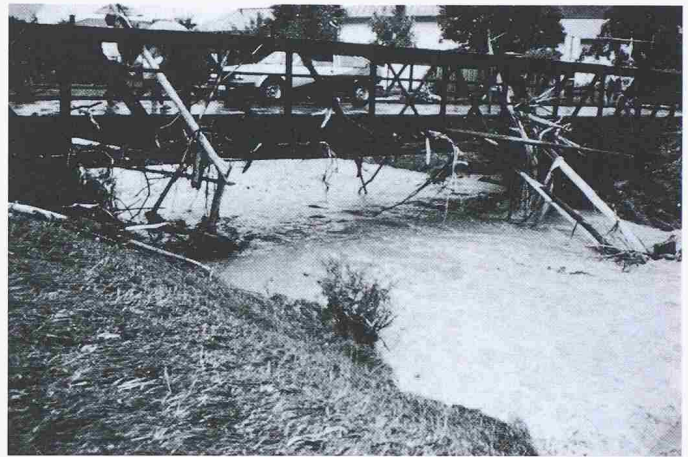
Bild 9. Brücke über die Alp nach dem Hochwasser 1984. Eine bergseitige Verschaltung hätte hier das Hängenbleiben von Holz verhindert (Foto Baudepartement des Kt. Schwyz, Abt. Wasserbau)
