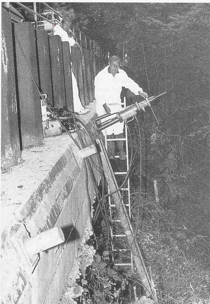
Bild 1. Leichte, tragbare Spannpresen erlauben Prüfungen auch an schwer zugänglichen Stellen
