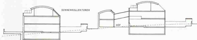
Schnitt
