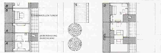
Dachgeschoss
