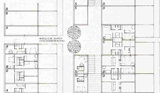
Dachgeschoss
