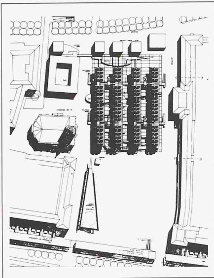
Links: Lageplan, rechts: Modellaufnahme, Altmarkt, Kreuzkirche
